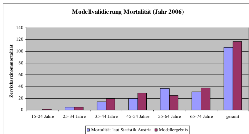
Abbildung 6.1-2: Modellvalidierung Mortalität
